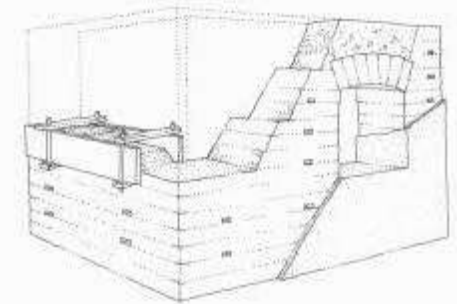
Vert fal szerkezete és készítése jámos zsuzuzattal (A kép forrása: www.sze.hu )
